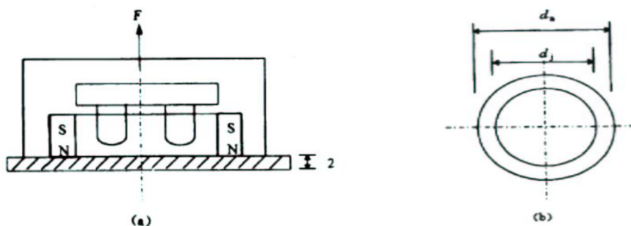
图2 磁钢的特性参数
