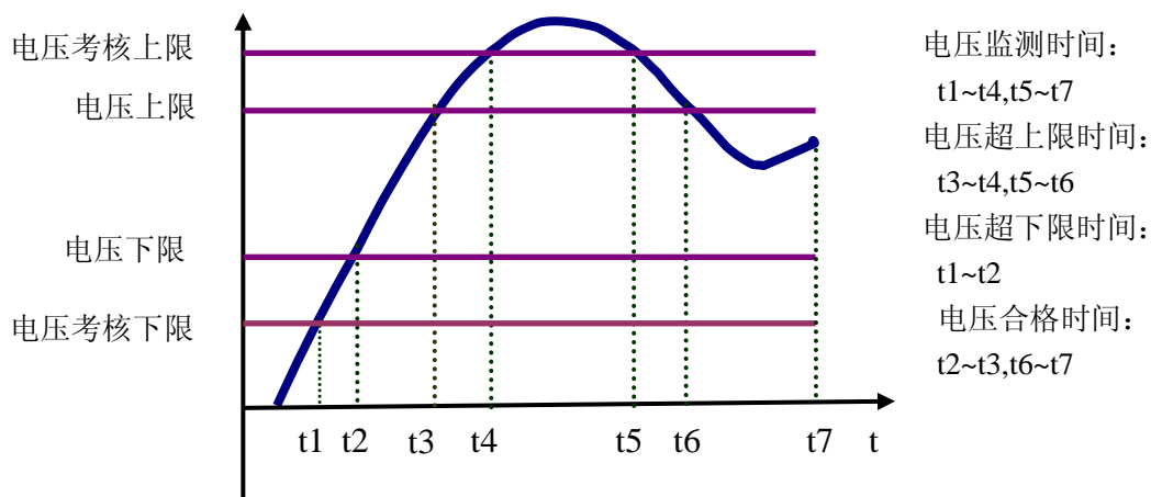
图 1 电压合格率判断示意图
